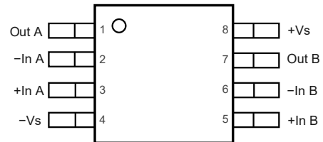
TPA5582
