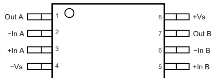
TPA5582
