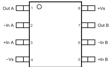
TPA5582
